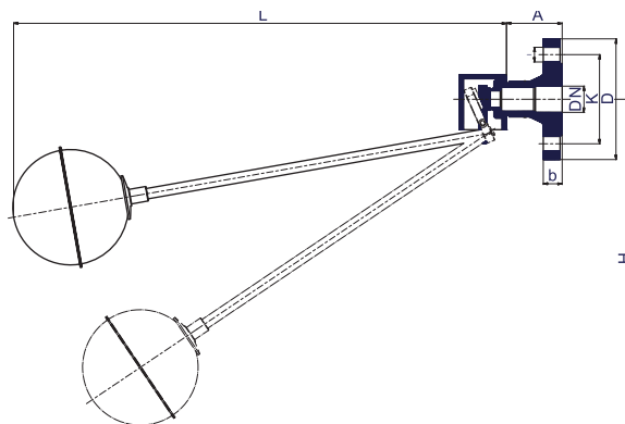
Фланцевое присоединение
