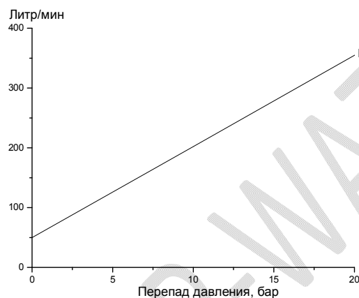
Диаграмма 1. Зависимость расхода от давления
