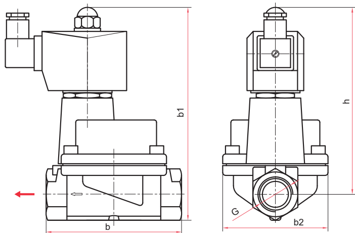
Габаритные и присоединительные размеры (мм), вес (кг)
